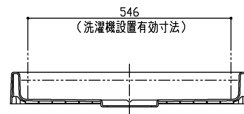
断面B-B
